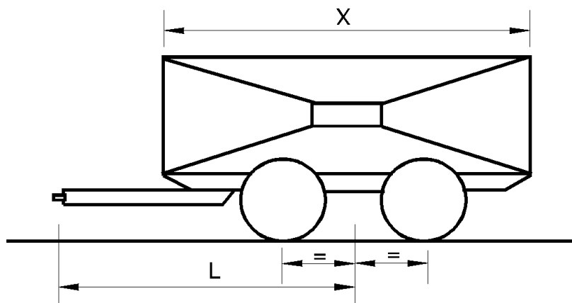
Rysunek 1 – Wymiary przyczepy z osią centralną
