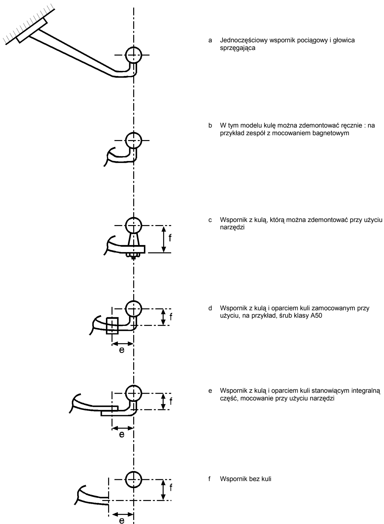
Rysunek 20 – Ułożenie wsporników kulowych
