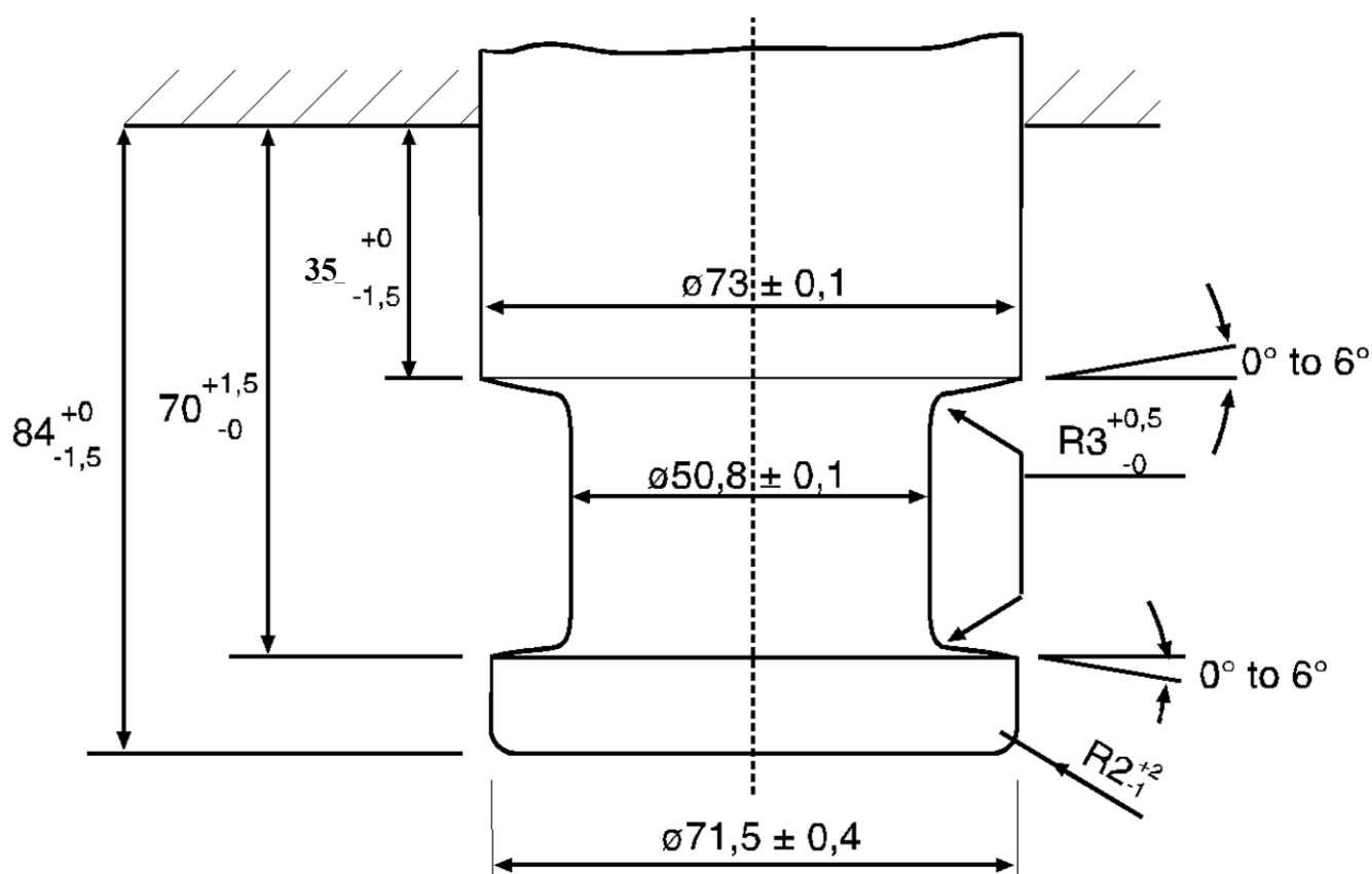
Rysunek 18 – Wymiary sworzni sprzęgu siodłowego klasy H50
