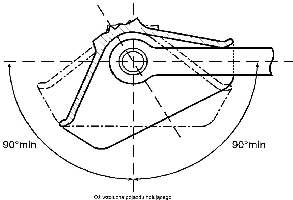
Rysunek 5 – Pozioma rotacja sprzężonego ucha dyszla pociągowego
