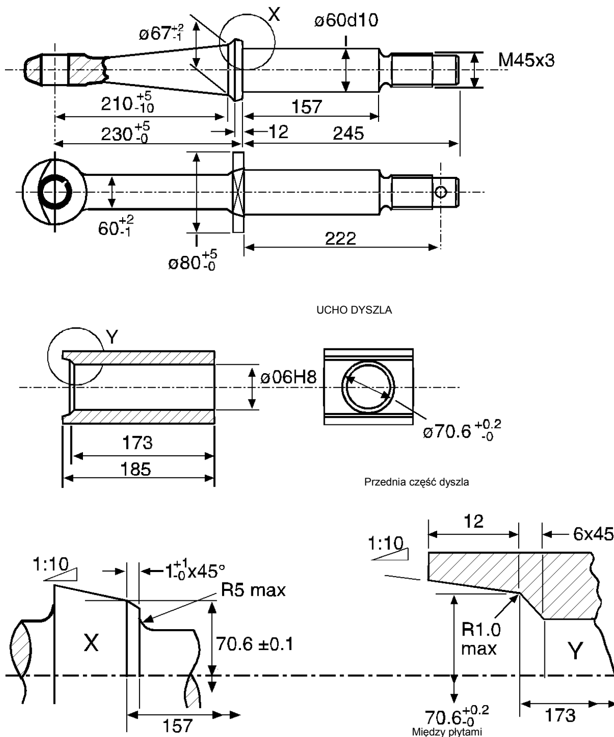
Rysunek 12 – Wymiary uch dyszla pociągowego klasy D50-B, pozostałe wymiary patrz Rysunek 11
