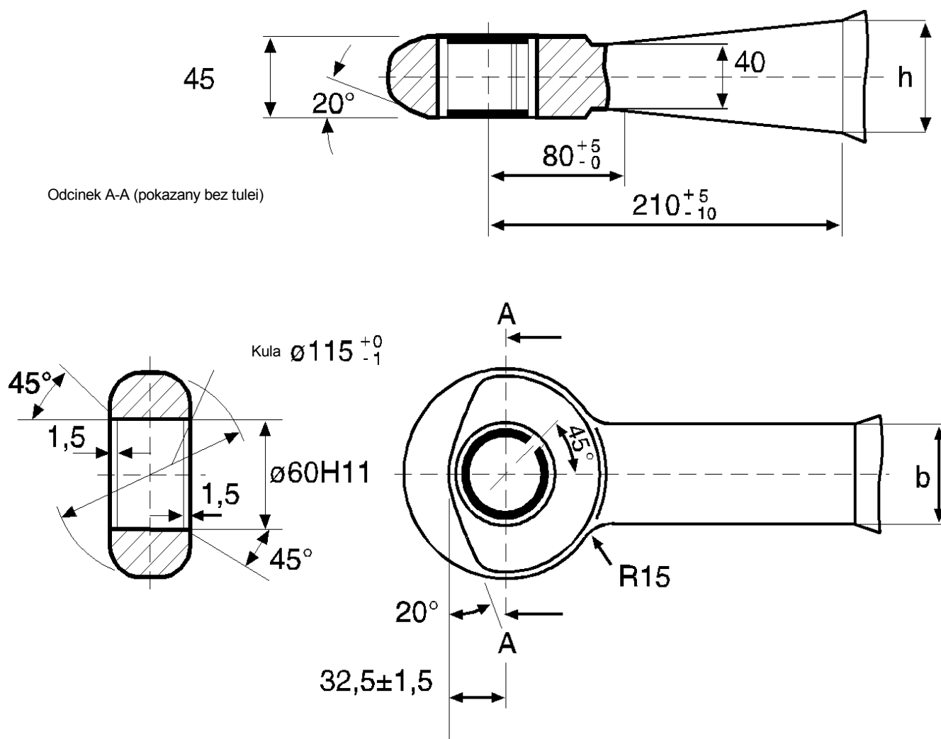
Rysunek 11 – Wymiary ucha dyszla pociągowego klasy D50-A i D50-X, patrz Tabela 6
