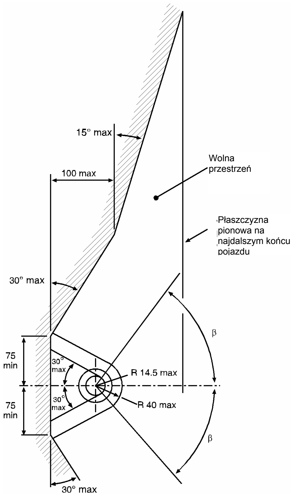
Rysunek 25(b) – Prześwit zaczepu kulowego – widok z góry
