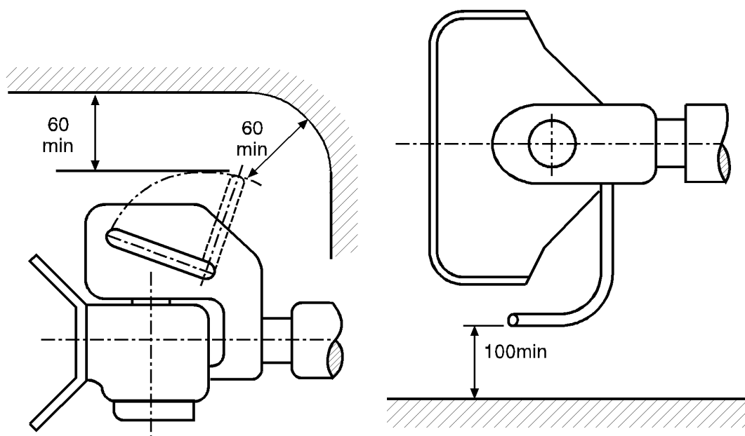
Rysunek 26 – Wolna przestrzeń wokół dźwigni ręcznej
