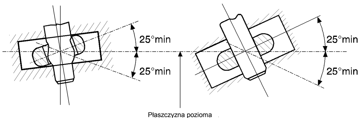
Rysunek 7 – Rotacja osiowa sprzężonego ucha dyszla pociągowego
