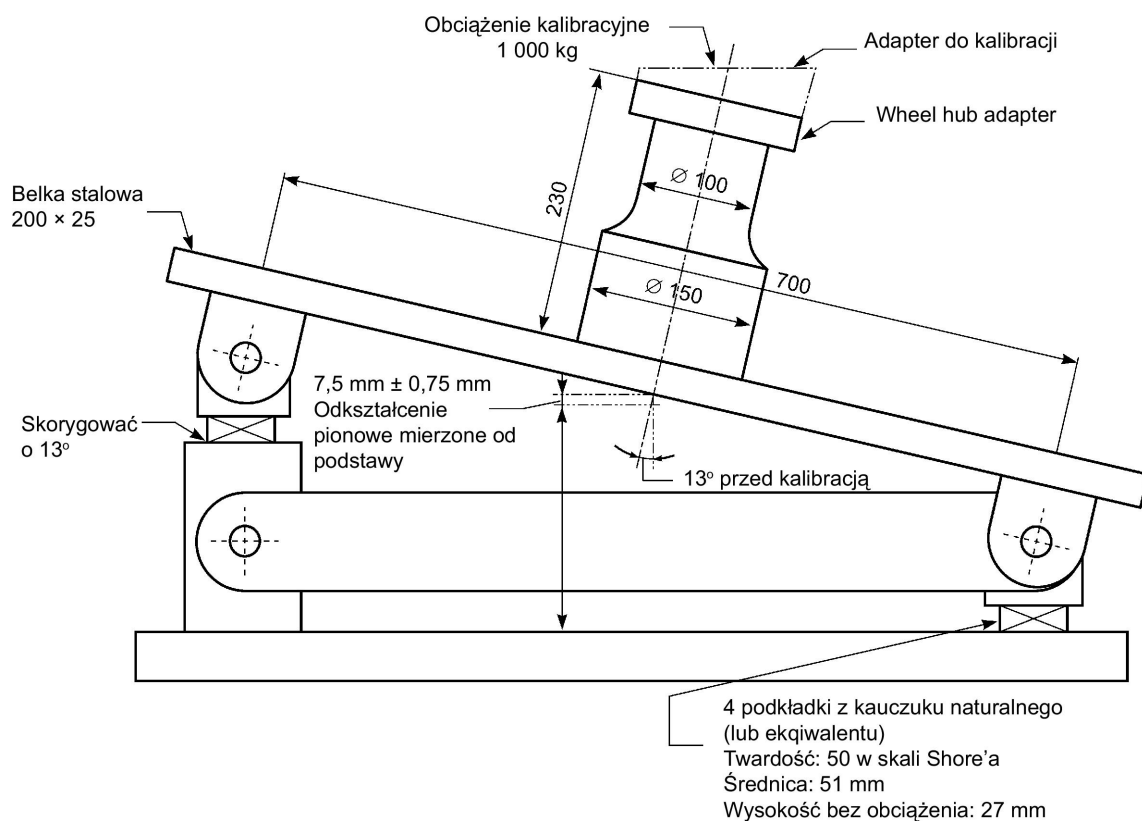
Rys. 2 – Przyłożenie obciążenia do środka mocowania koła
