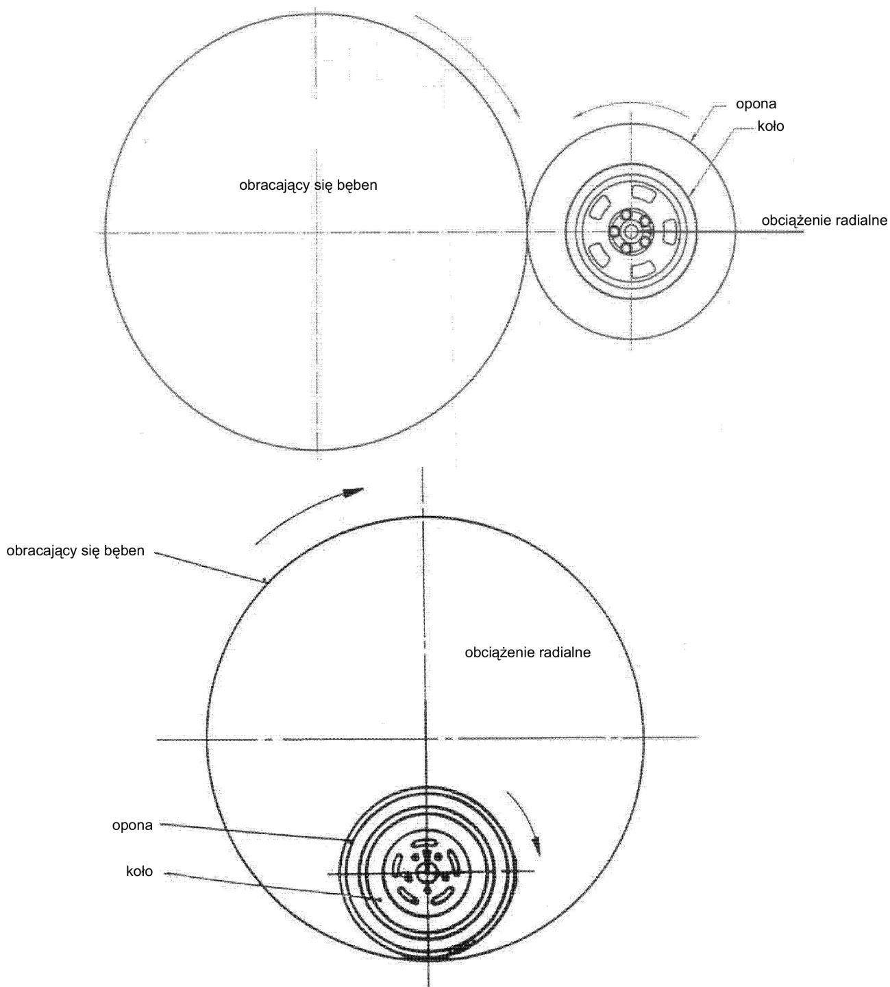
Przykładowe urządzenie do badań odporności na toczenie
