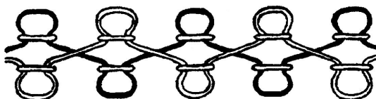
Rysunek 9 Splot interlokowy
